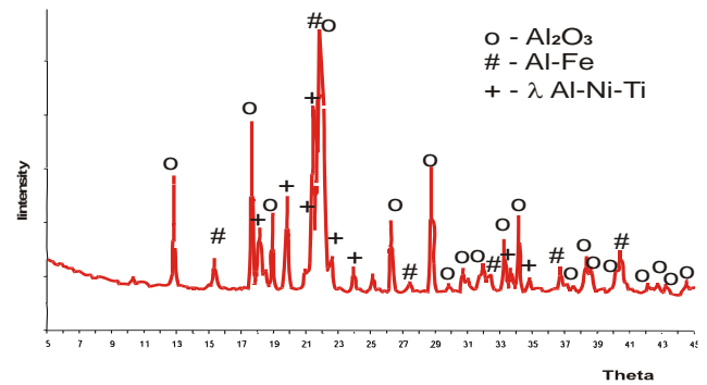
Fig. 3. Diffraction pattern of NiCr-FeAl-TiAl-Al 2 O 3 composite powders Rys. 3. Dyfraktogram proszku kompozytowego NiCr-FeAl-TiAl-Al 2 O 3
